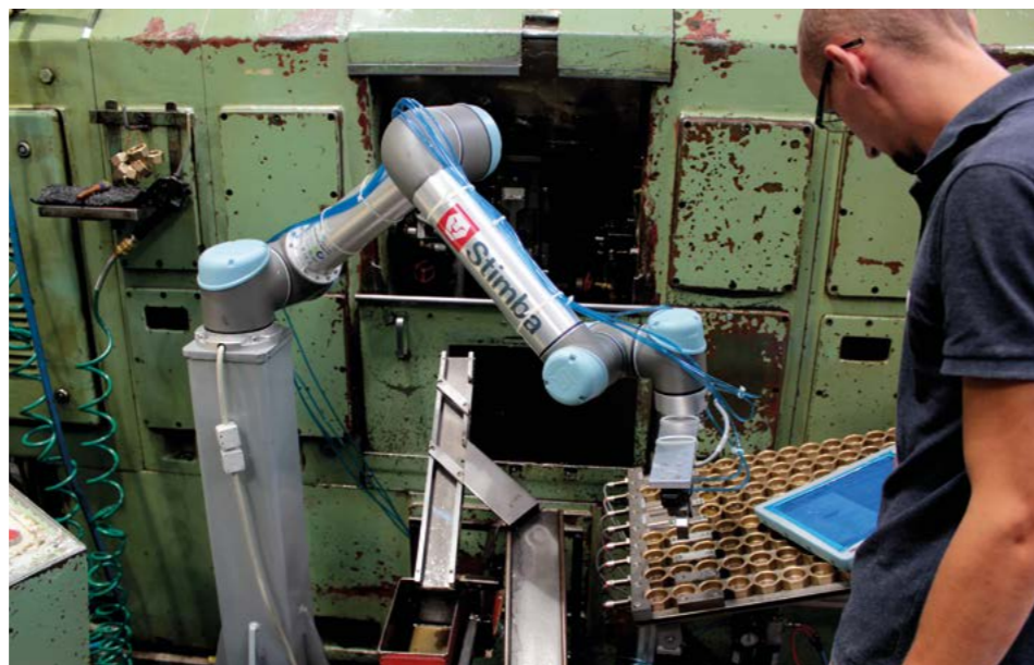
Stroj VAGON čaká na čiastočnú opravu, robot je úplne nový. Pochádza z Čiech.
