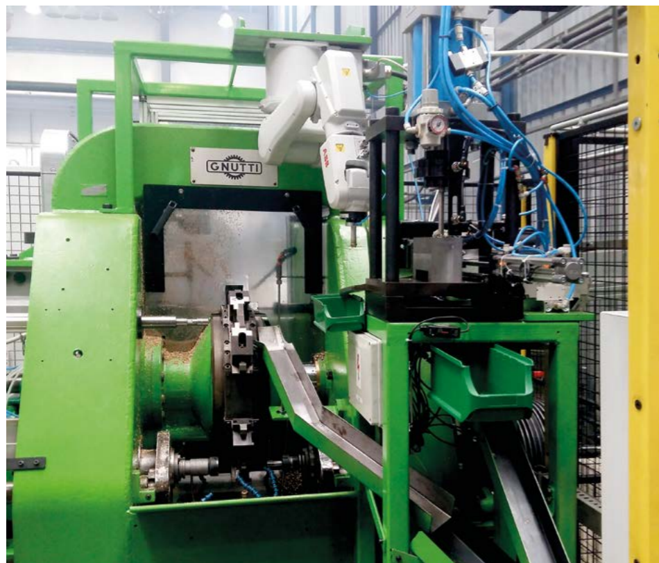
Stroj Gnutti je po generálnej oprave, robot ABB spoločne s vibračným zásobníkom je kompletne nový. Pochádza z Talianska.
